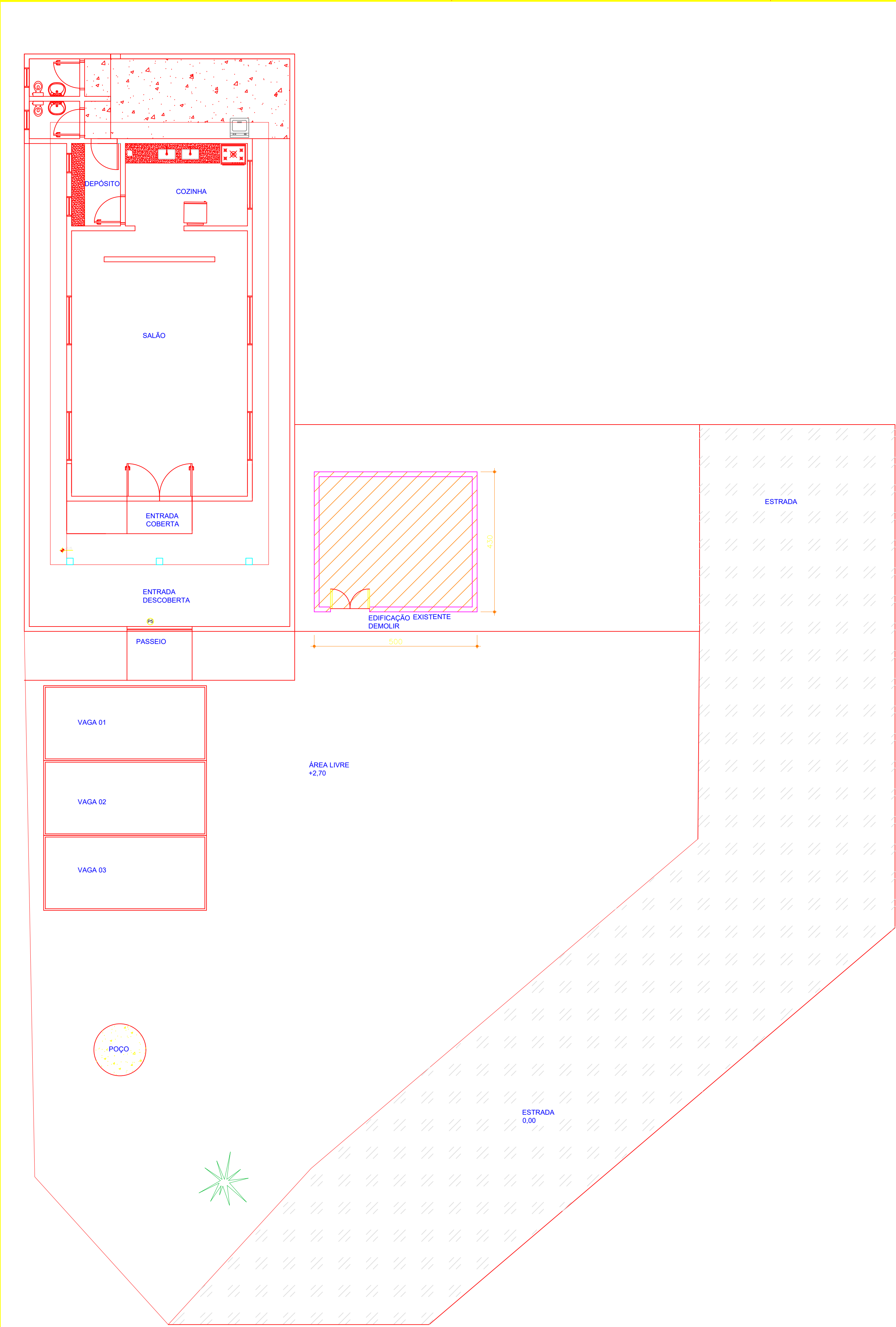
PLANTA DEMOLIR ESCALA 1/75 OBS: demolir edificação atual que abriga tanque — 21,50m² Legenda Alvenaria a demolir
