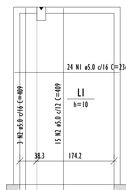
ARMAÇÃO POSITIVA DAS LAJES DO PAVIMENTO NÍVEL +300 ESCALA 1:50
