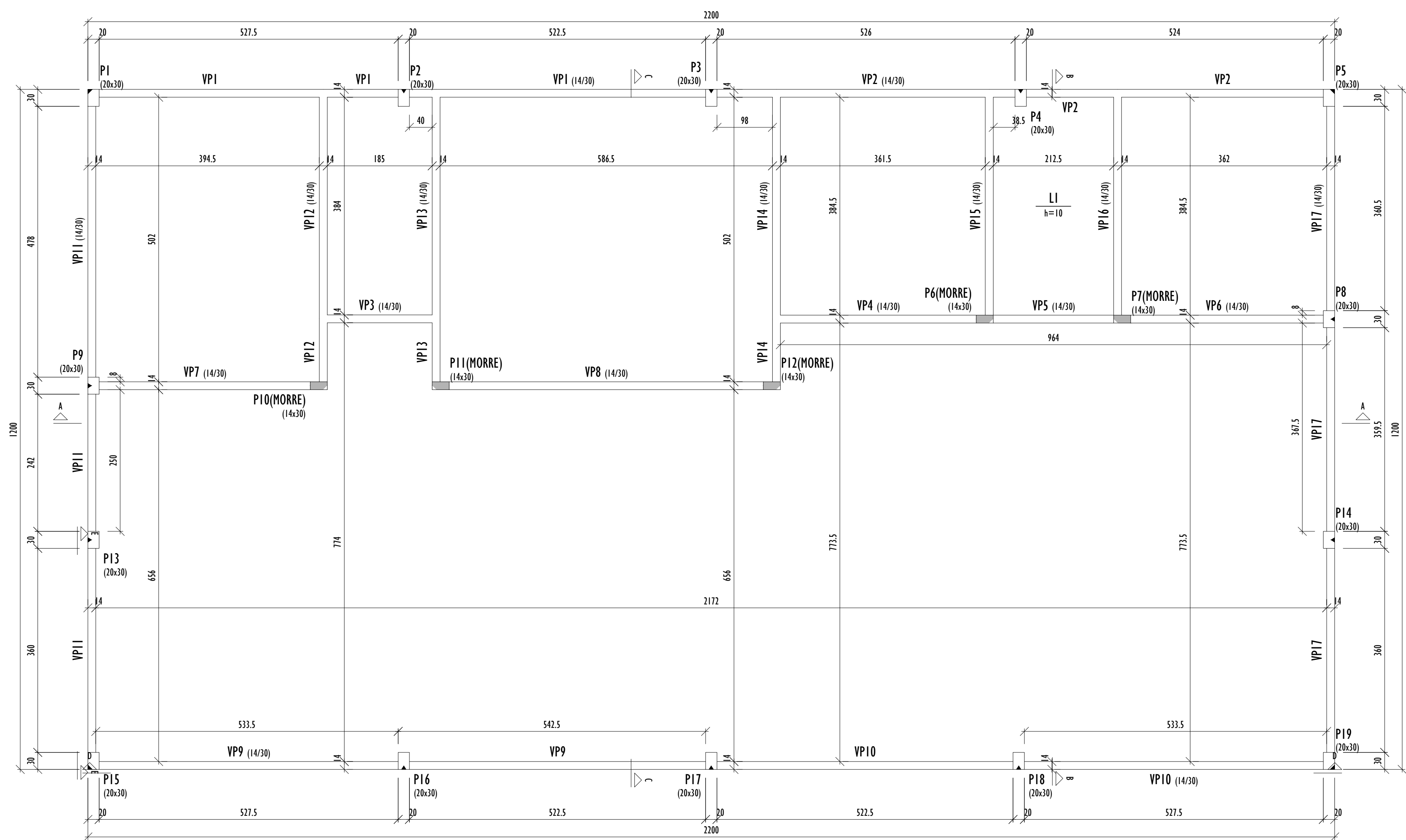
FORMA DO PAVIMENTO NÍVEL +300 (NÍVEL 500) ESCALA 1:50
