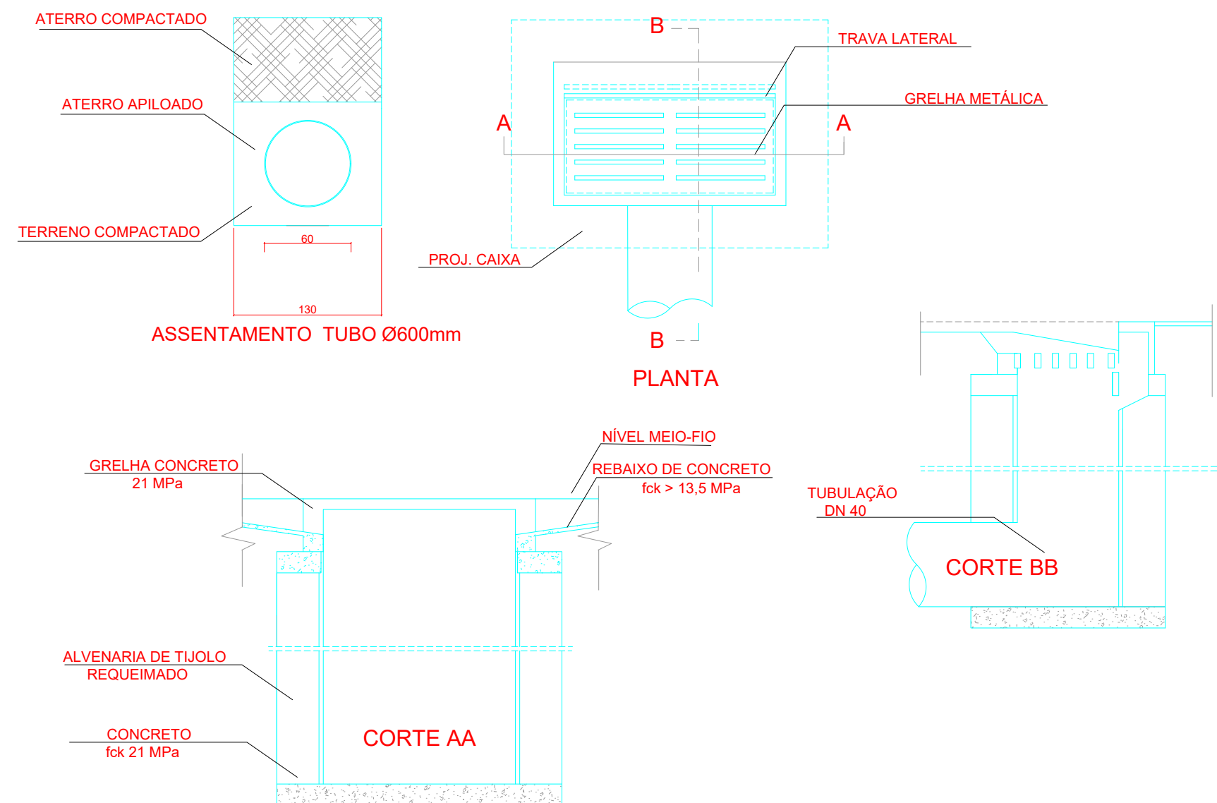
DETALHES CAIXAS DRENAGEM SEM ESCALA
