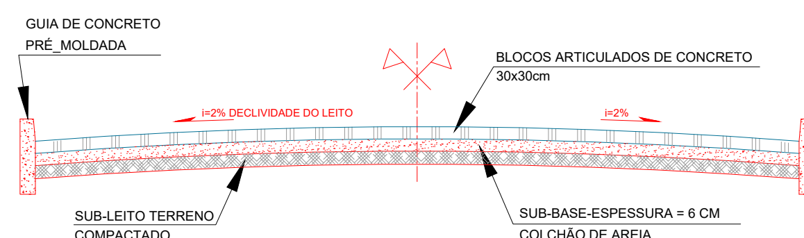
PERFIL TRANSVERSAL SEM ESCALA
